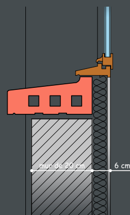
Détail appui de 28
