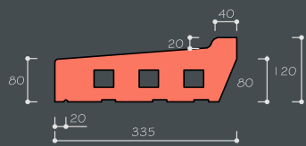
Appui de 33
