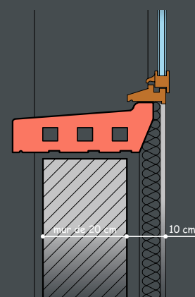
Détail appui de 33 Mise en œuvre identique pour appui de 37
