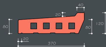
Appui de 37
