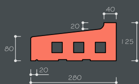
Appui de 28
